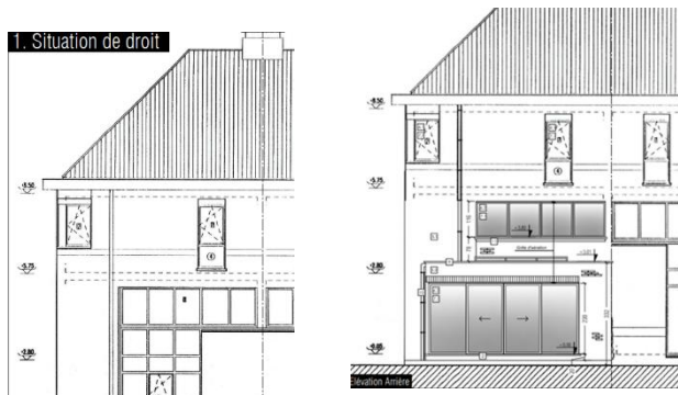
Façade arrière donnant sur le site classé : état existant et projeté – documents extraits du dossier de demande
