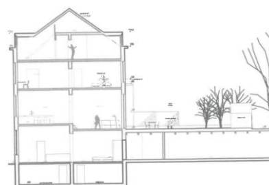
Snede van de projectsituatie. Beeld uit het aanvraagdossier
