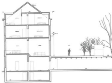
Snede van de bestaande situatie. Beeld uit het aanvraagdossier
